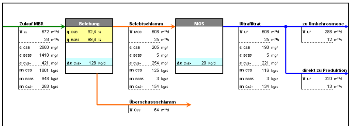
Abbildung 6: Bilanzkreis Biologie und MBR - Betrieb des 1. Anlagenabschnitt
