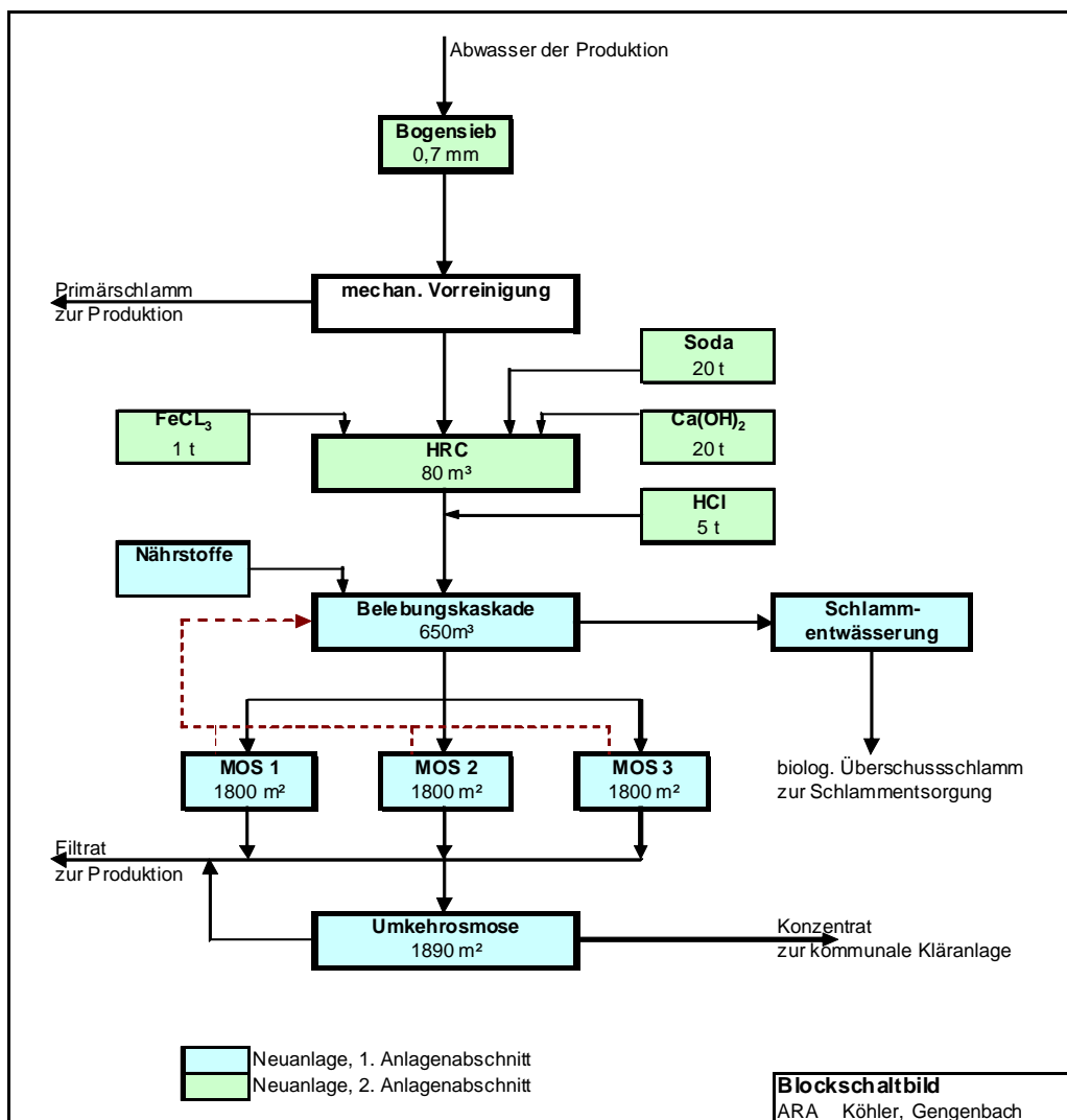
Abbildung 2: Blockschartbild der Verfahrensstufen
