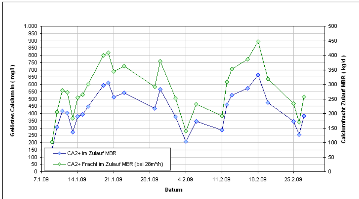
Abbildung 5: Calcium Zulaufkonzentration und Tagesfracht des MBR Anfang 2009
