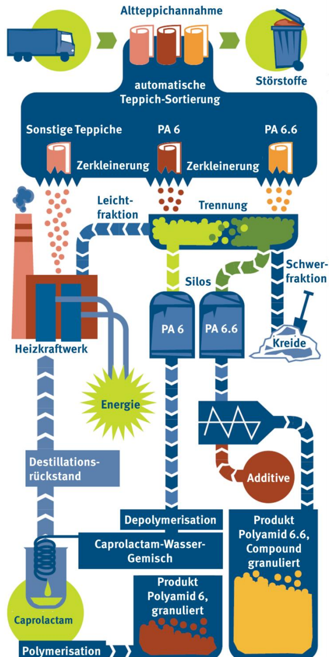
Abbildung 2: Verfahrensschema für Recycling von Polyamid-Altteppichen
